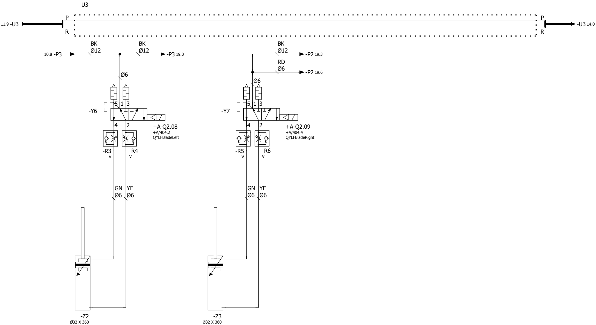
LAME DE PLIAGE GAUCHE
