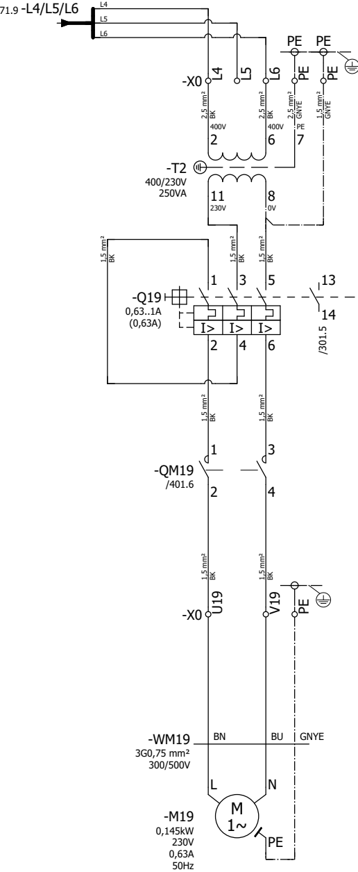
MOTEUR, ASPIRATION, ENTREE
