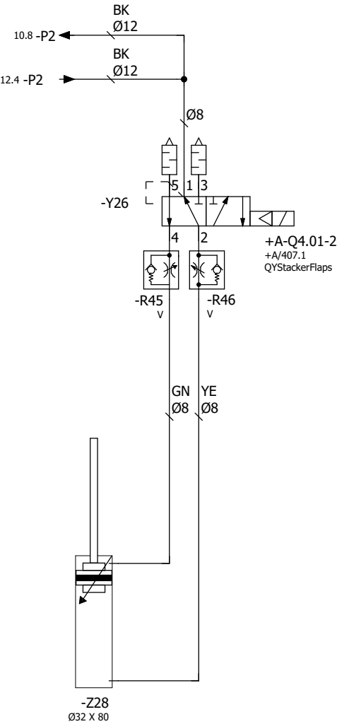
VOILETS EMPILEUR FERMER DROITE
